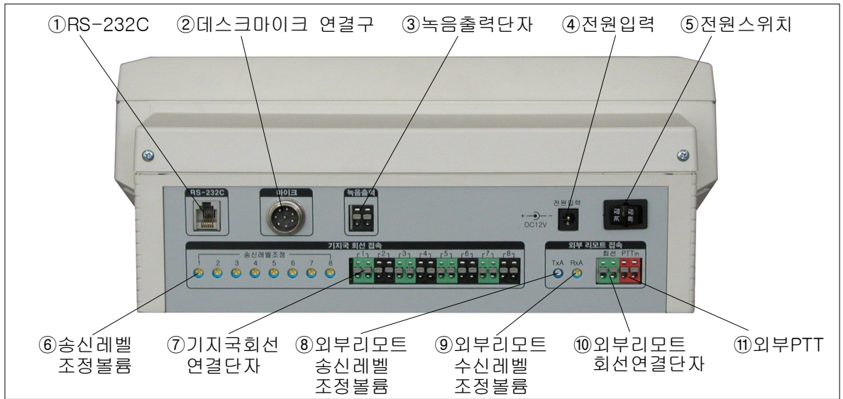
그림3 다채널원격제어장치(MRT-800D)의 외형(후면)
