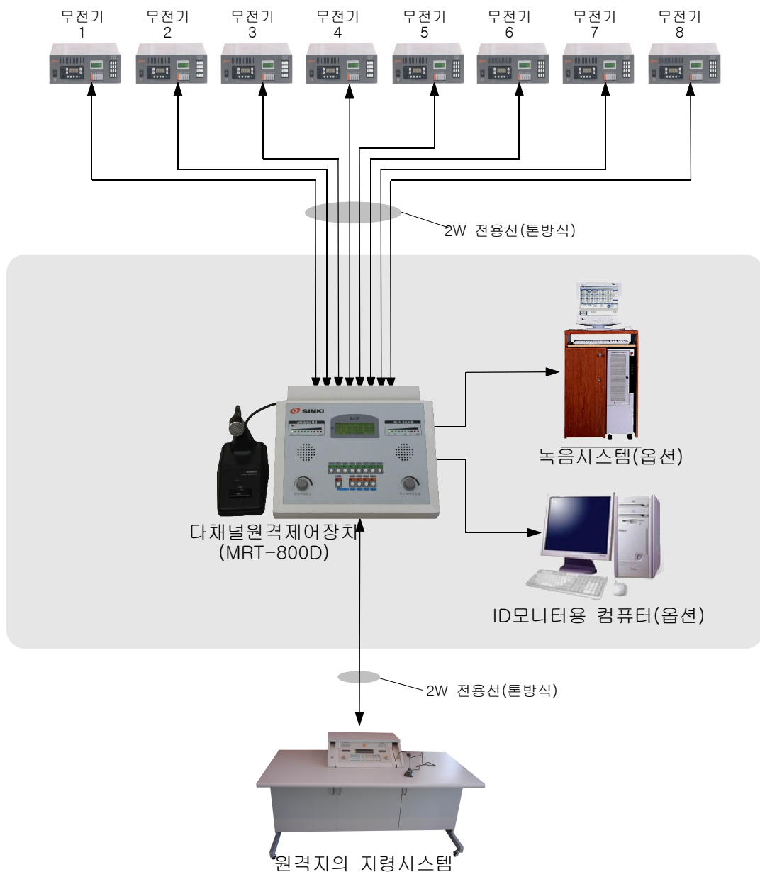
그림1 시스템 구성도
